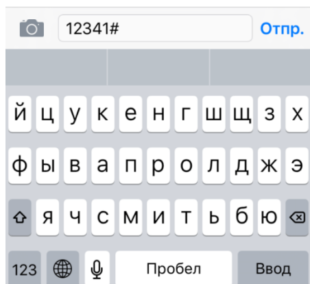
Рис. 1.7. Отправка сообщения
